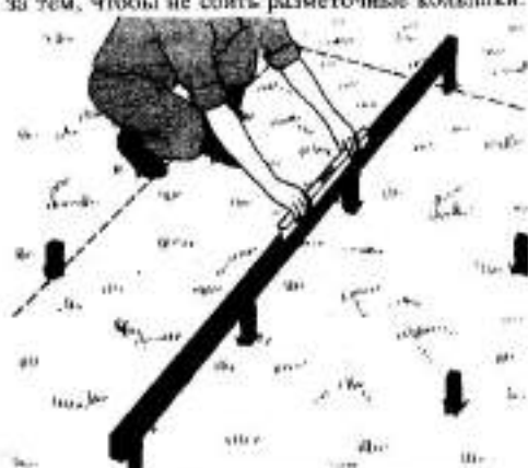
4 Выровняйте все основание с помощью промежуточных кольшачков, установленных на расстоянии 1,5 м друг от друга по всей поверхности дворика, так, чтобы их высота совпадала с высотой кольшачков, расположенных по периметру.
