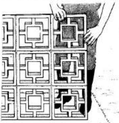
2 Выложите первую стенку из ажурных блоков, начиная от первого крайнего столба. Стенка должна быть высотой в три ряда блоков.
