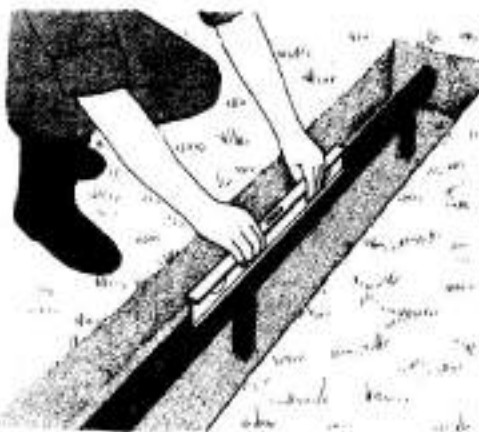
5 Вбейте кольшки в дно траншеи для определения в дальнейшем высоты укладываемого слоя бетона. Проверьте, все ли они находятся на одном уровне.
