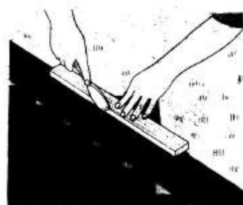
4 Разметьте стамеской блоки, которые необходимо обрезать, установив их над местом для укладки.
