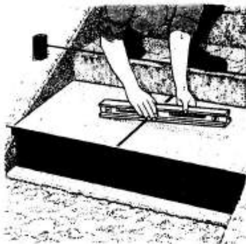
7 Обеспечьте уклон, необходимый для стока дождевой воды, слегка наклонив ступень вперед.
