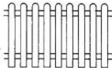
Изгороди из вертикальных штакетинок и горизонтальных перекладин используют для ограждения палисадника и окрашивают белой краской.
